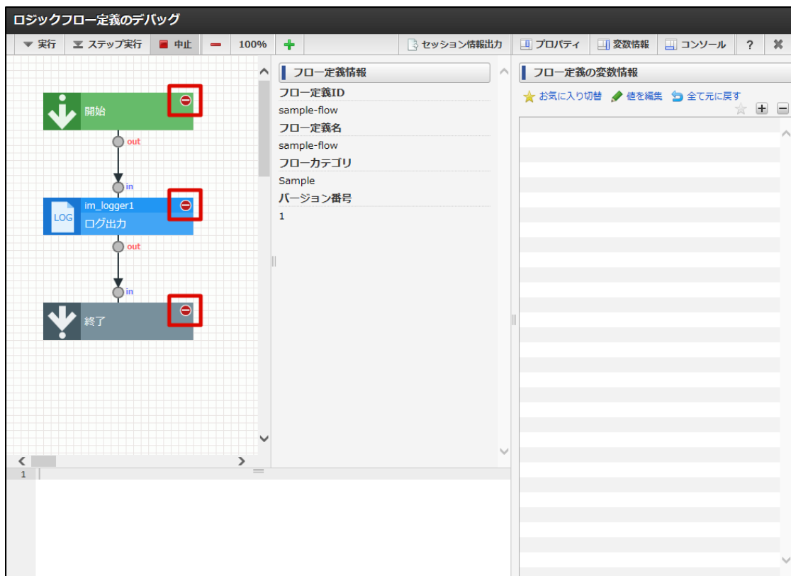
図：複数のブレークポイントを設定したフロー
