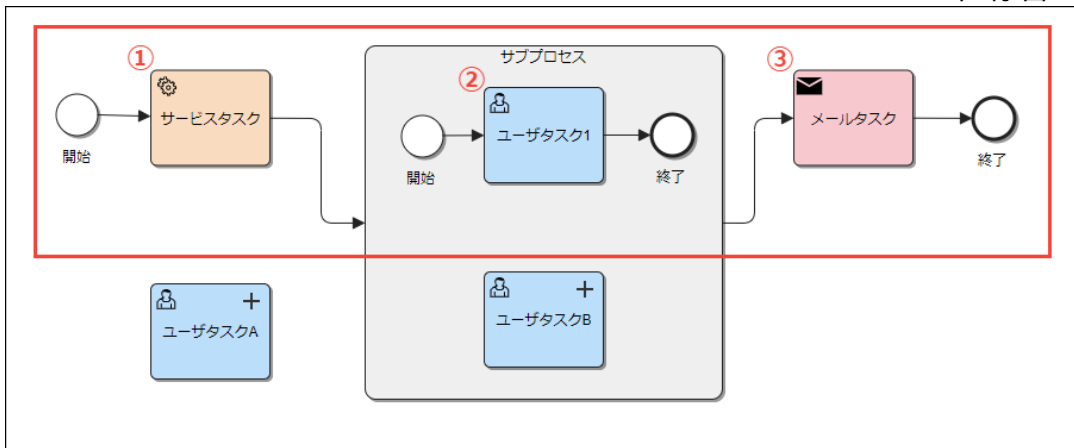
図：プロセスインスタンスの実行の流れ
